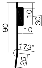
SEZIONE B
