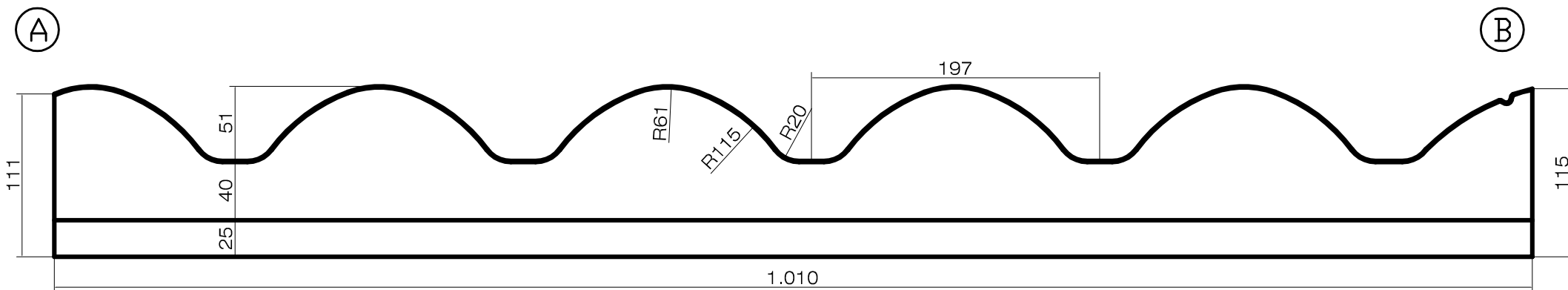
SEZIONE A
