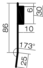
SEZIONE A
